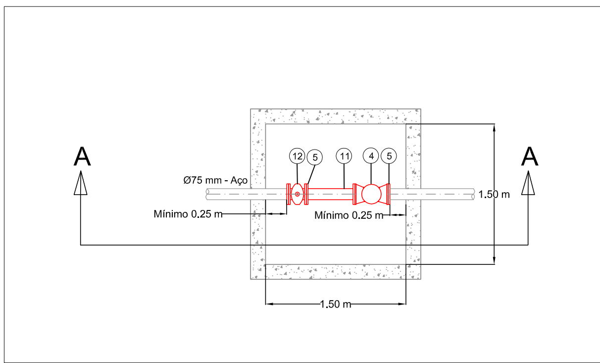
MACROMEDIDOR ULTRASSÔNICO - MM 01
