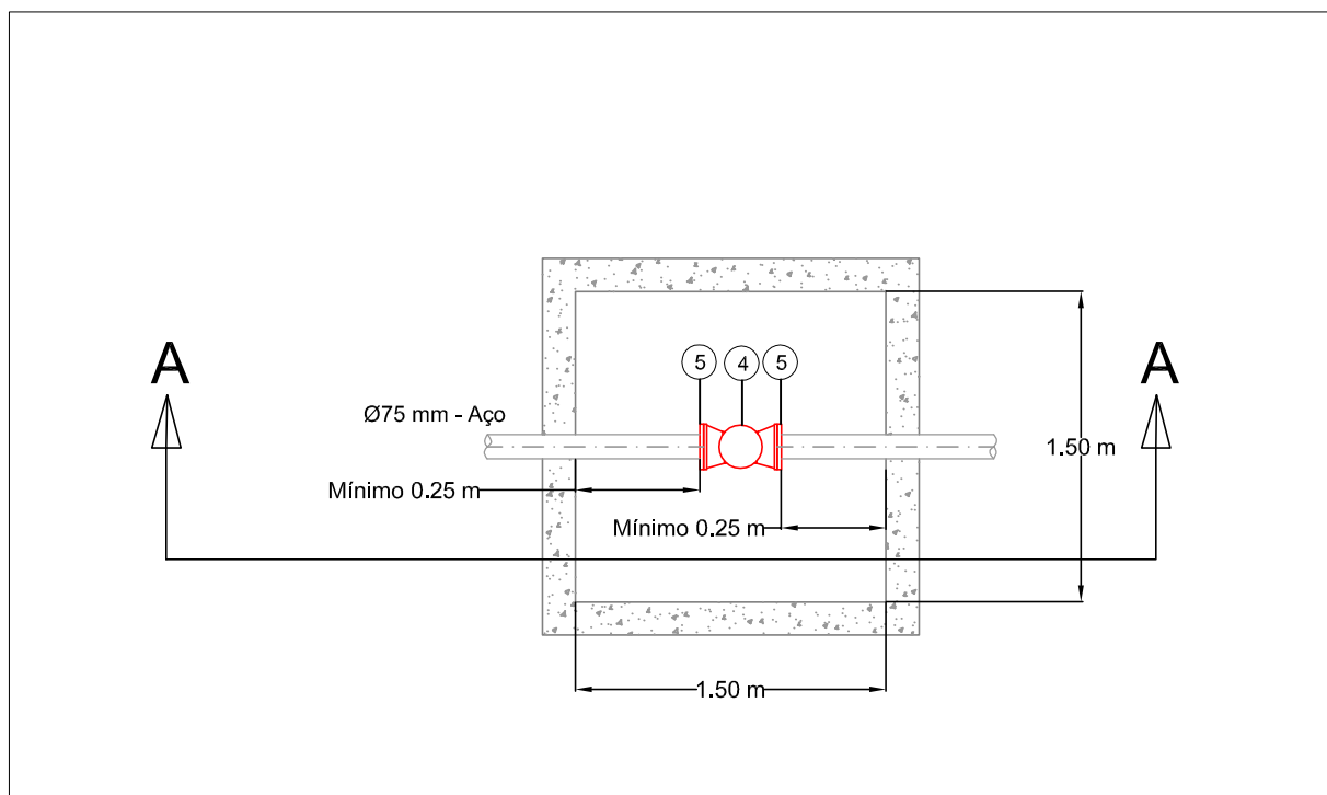
MACROMEDIDOR ULTRASSÔNICO - MM 05
