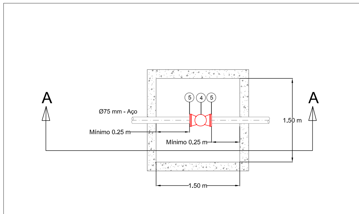
MACROMEDIDOR ULTRASSÔNICO - MM 07
