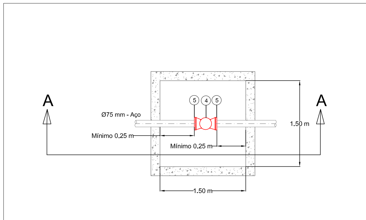
MACROMEDIDOR ULTRASSÔNICO - MM 08
