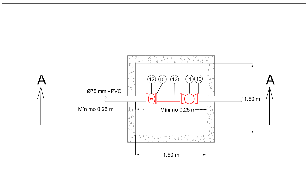
MACROMEDIDOR ULTRASSÔNICO - MM 02
