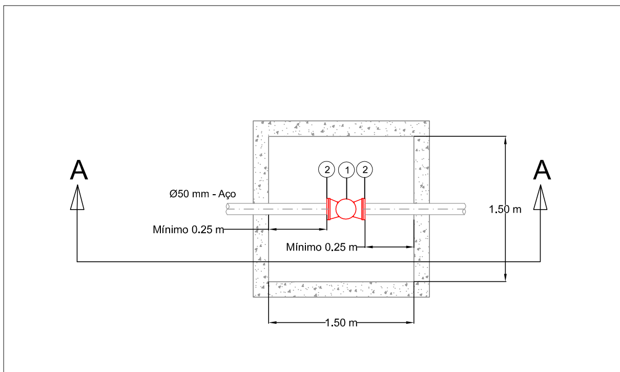
MACROMEDIDOR ULTRASSÔNICO - MM 06
