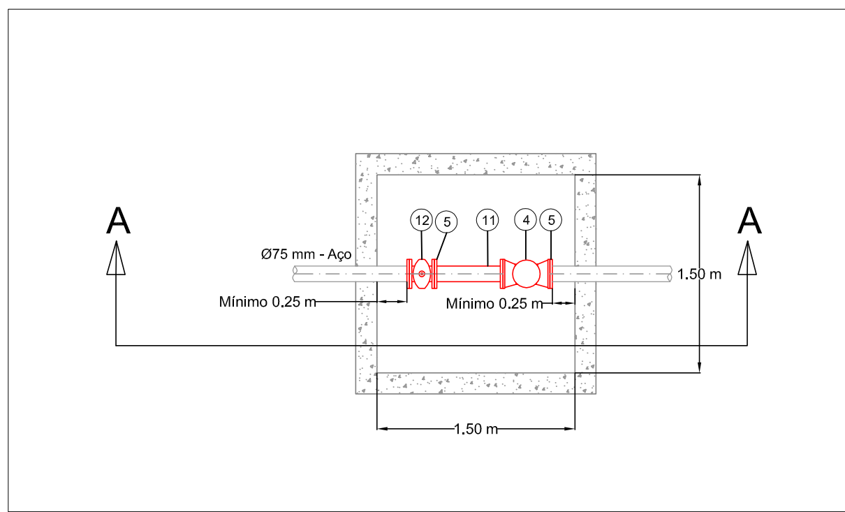
MACROMEDIDOR ULTRASSÔNICO - MM 04
