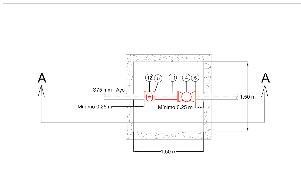
MACROMEDIDOR ULTRASSÔNICO - MM 03
