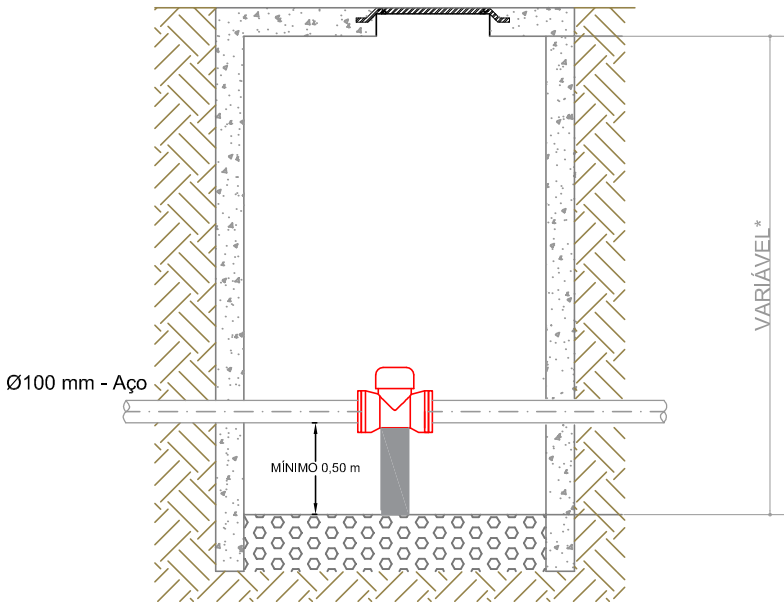
LISTA DE MATERIAIS PARA IMPLANTAÇÃO DOS MACROMEDIDORES DE VAZÃO - POÇOS PROFUNDOS
