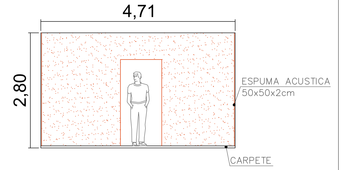
VISTA A - SALA ACÚSTICA (PERFIL) S/ ESC.
